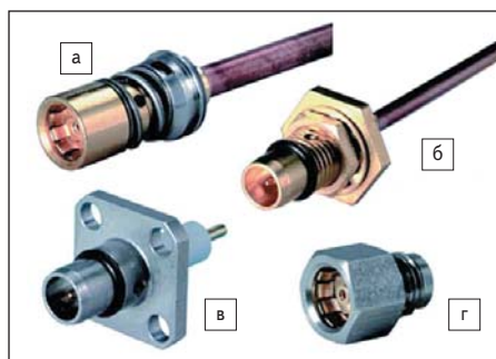
Рис. 6. Соединители BMA: а) розетка проходная для полужесткого кабеля; б) вилка приборно-кабельная для полужесткого кабеля; в) ввод энергии — вилка панельная фланцевая; г) ввод энергии — розетка резьбовая
