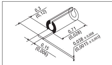
Рис. 9. Скользящий контакт 73-Z-0-0-204 (в скобках — размеры в дюймах)
