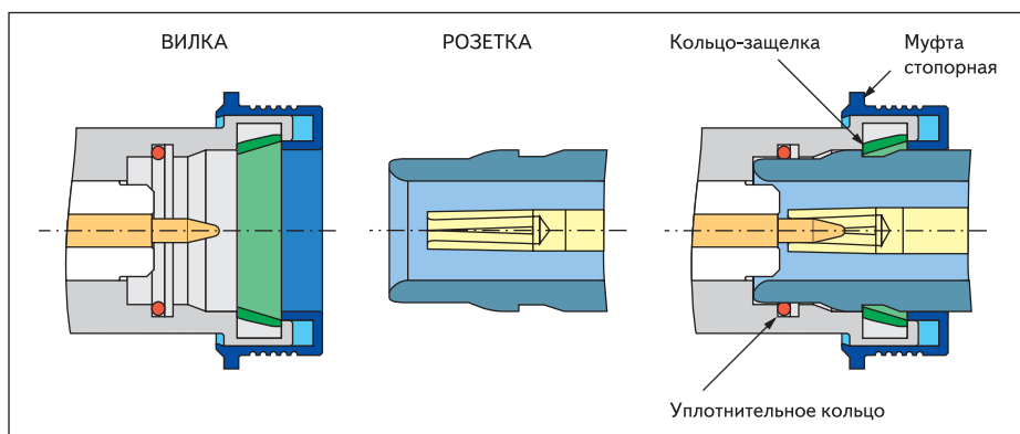
Рис. 10. Конструкция вилки и розетки соединителей QN
