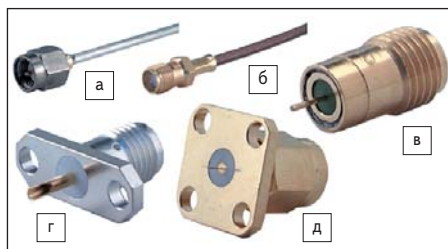
Рис. 1. Соединители SMA:
