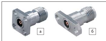
Рис. 7. Вводы энергии PC3.5 — розетка со сменными контактами: а) с квадратным фланцем; б) с прямоугольным фланцем
