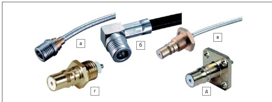
Рис. 4. Соединители QMA: а) вилка прямая для полужесткого кабеля; б) вилка угловая для гибкого кабеля; в) розетка приборно-кабельная; г) ввод энергии — розетка; д) ввод энергии панельный фланцевый
