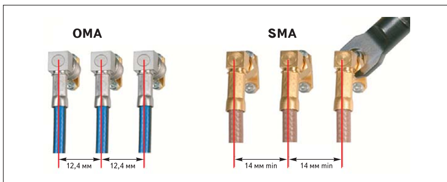
Рис. 3. Сравнение соединителей QMA и SMA (предоставлено фирмой Huber+Suhner)
