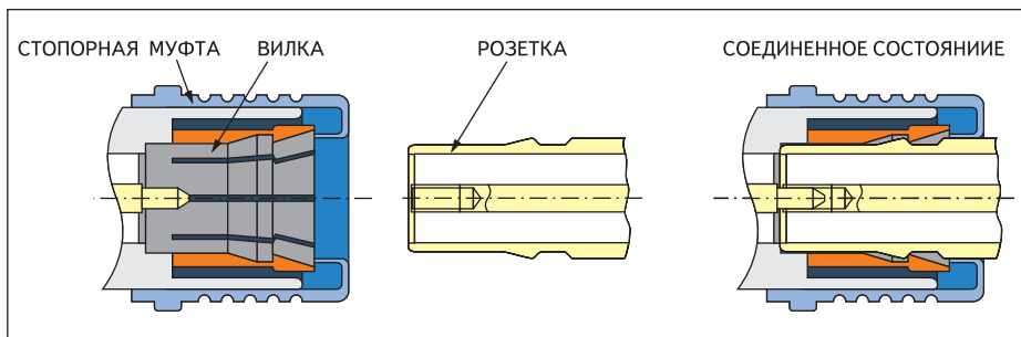
Рис. 2. Конструкция вилки и розетки QMA (предоставлено фирмой Huber+Suhner)
