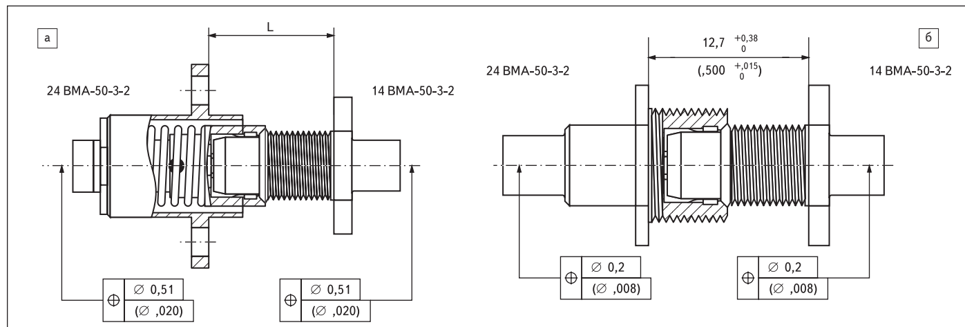
Рис. 5. Соединители BMA: а) фиксированная конфигурация (Rigid mounting); б) плавающая конфигурация (Float mounting)
